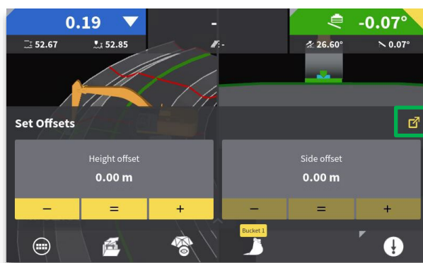
Step 2: Press the expansion button.
